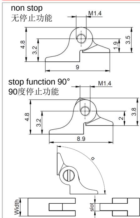
Profile: A nickel silver- 白铜A型
