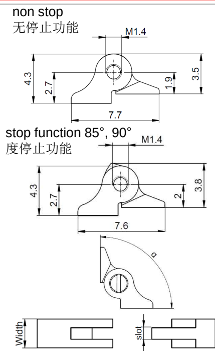
Profile: B nickel silver- 白铜B型
